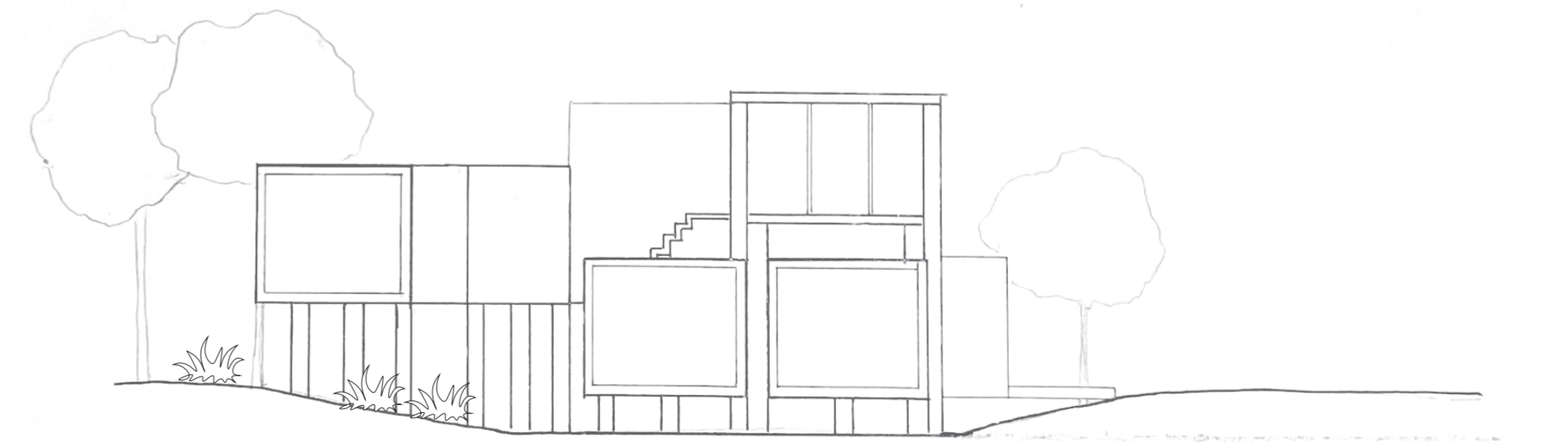
西立面図 1/100
