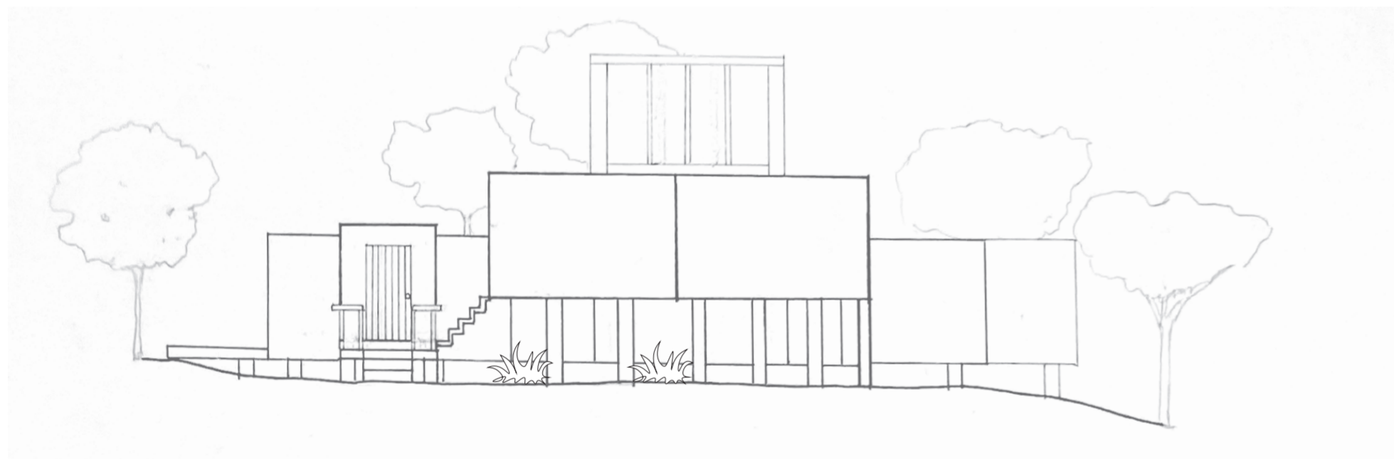
北立面図 1/100
