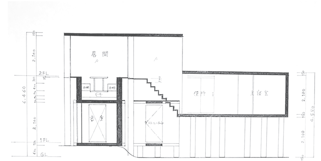
A-A 断面図 1/100
