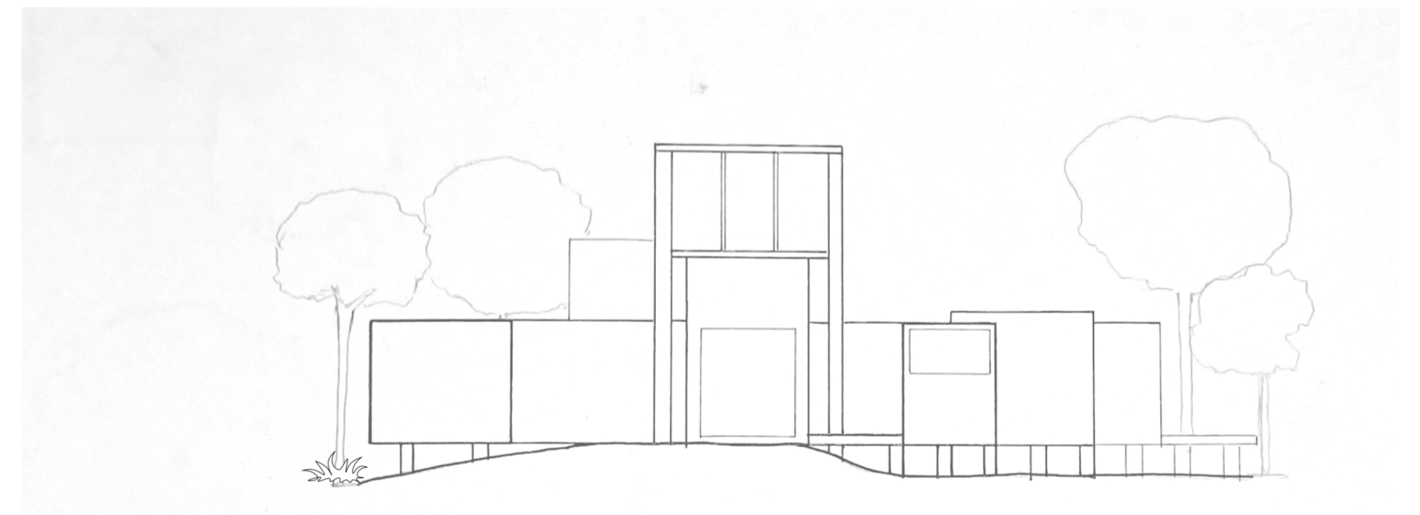
南立面図 1/100
