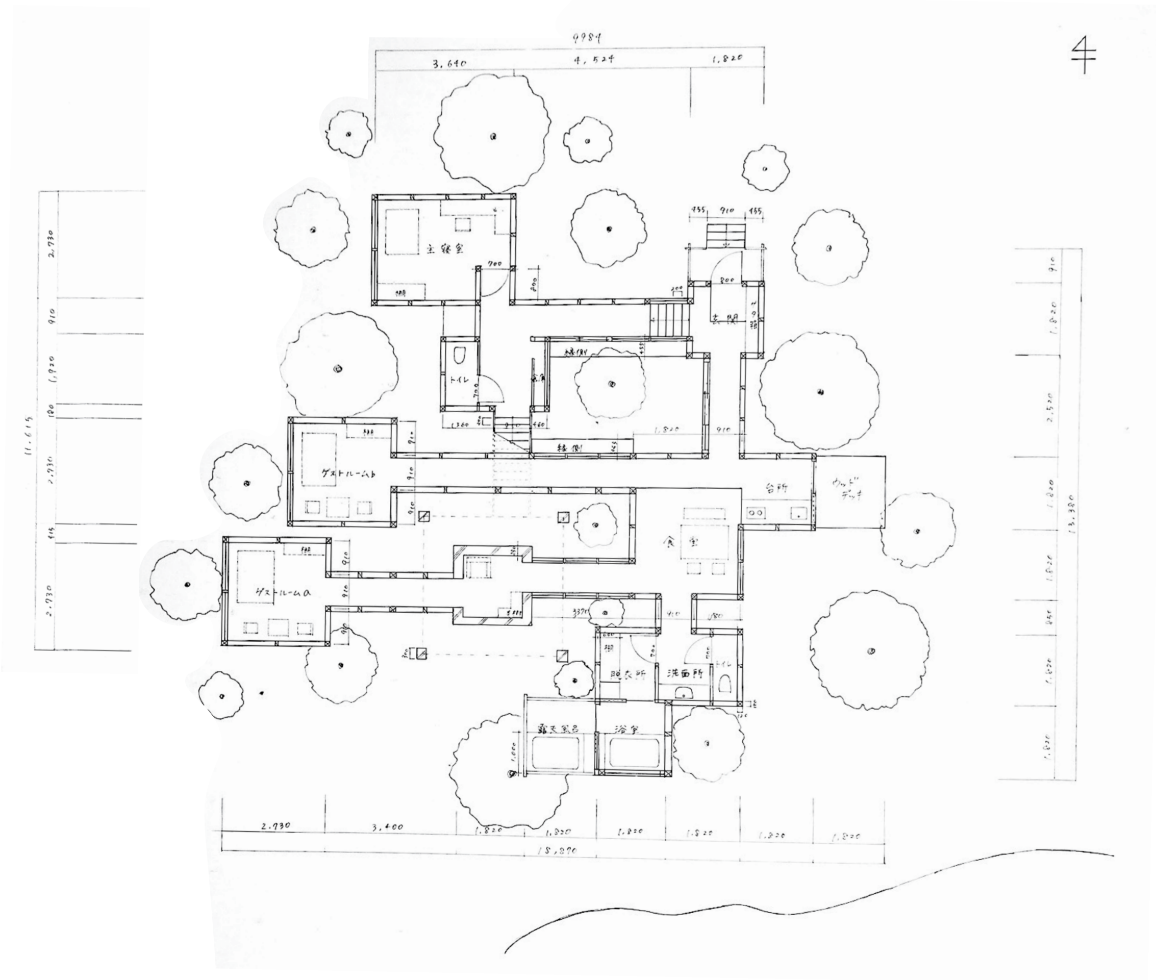
1 階平面図 1/100
