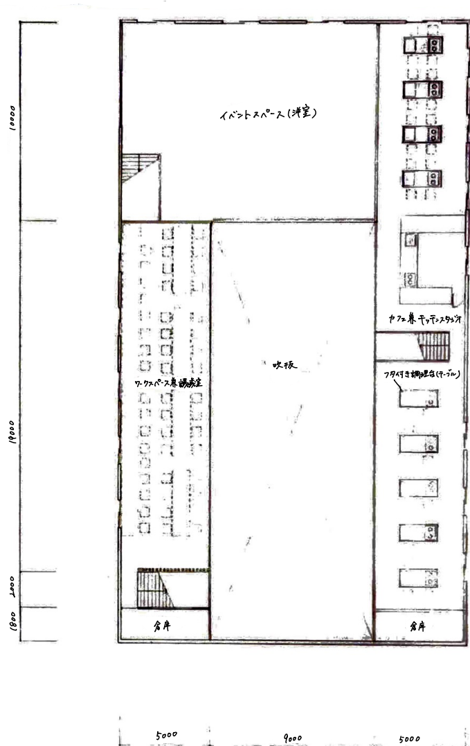
2F平面図 S=1:100
