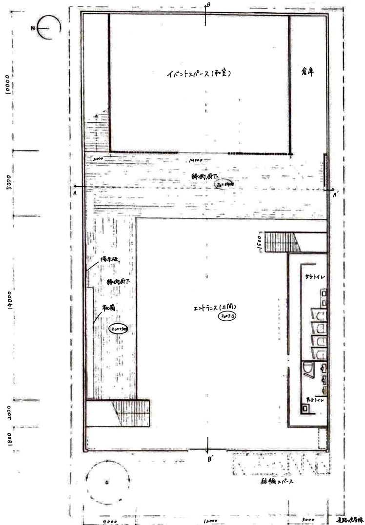
1F平面図 (和室) S=1:100
