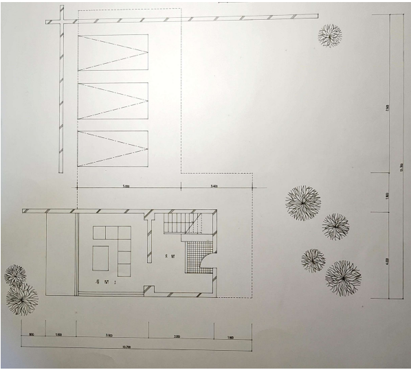
1階平面図
