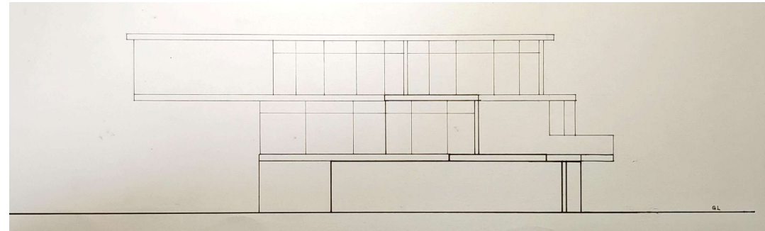
北立面図
